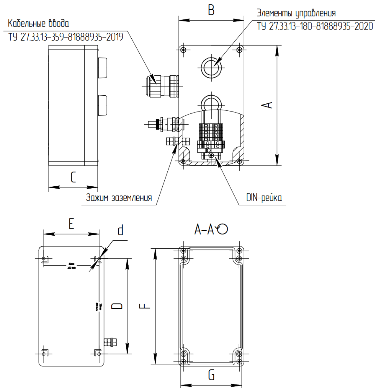
Рис. А1. Конструкция взрывозащищенных постов управления серии ПКВ, моделей: ПК МК Ехе-П-XXX... Х, ПКВ МК Ехі-П-XXX... Х из полиамида.
