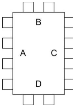
Рис. 1. Схема расположения вводов или отверстий в корпусе ПКВ МК Exe-II-XXX... X, ПКВ МК Exi-II-XXX... X.
