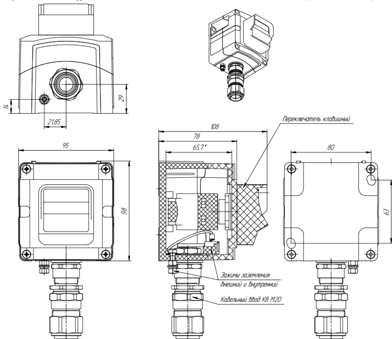
Рис. А2. Конструкция взрывозащищенных постов управления серии ПКВ стандартной комплектации, моделей: ПК МК Exe-П-101009 (П42), ПКВ МК Exi-П-101009 (П42) из полиамида.
